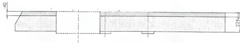
局部视图a(悬砵安装图) 比例: 1:3
