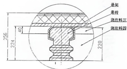
局部视图a(悬砵安装图) 比例: 1:3
